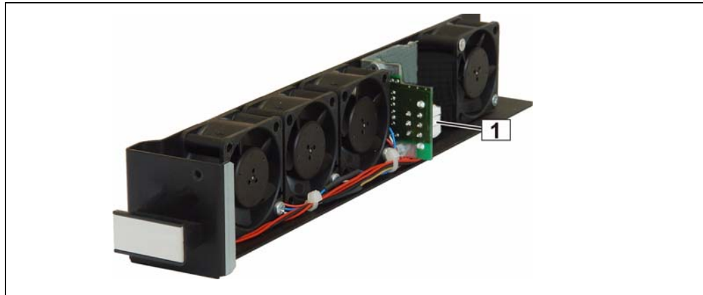
Figure 4: Lüftereinschub
