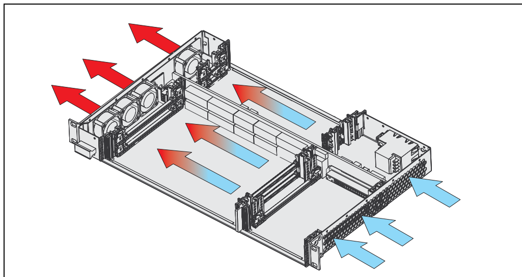
Figure 5: Entwärmung
