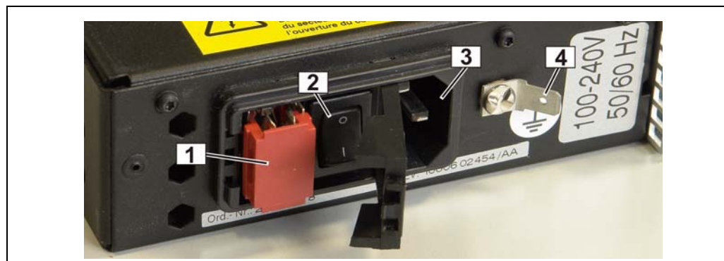
Figure 2: Netzeingangsmodul
