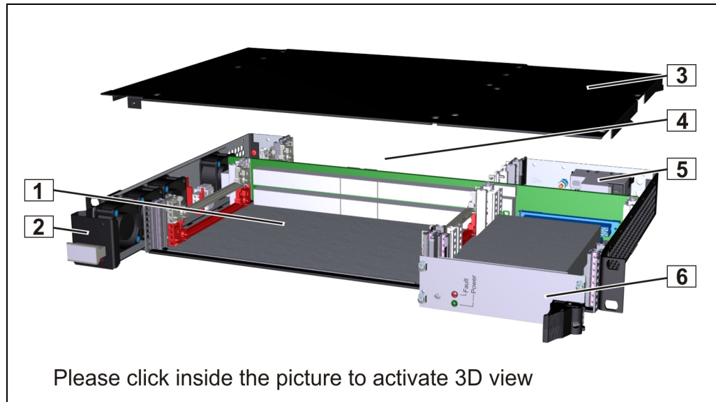
Figure 1: Einschubsystem Übersicht
